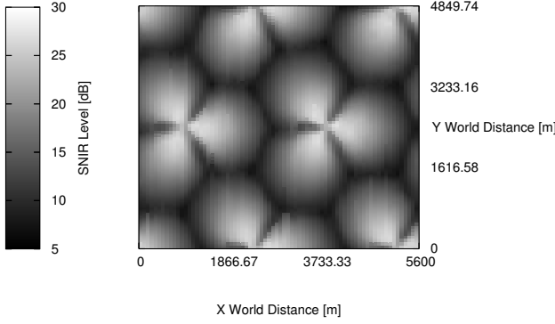
Fig. 9. SNIR map.
