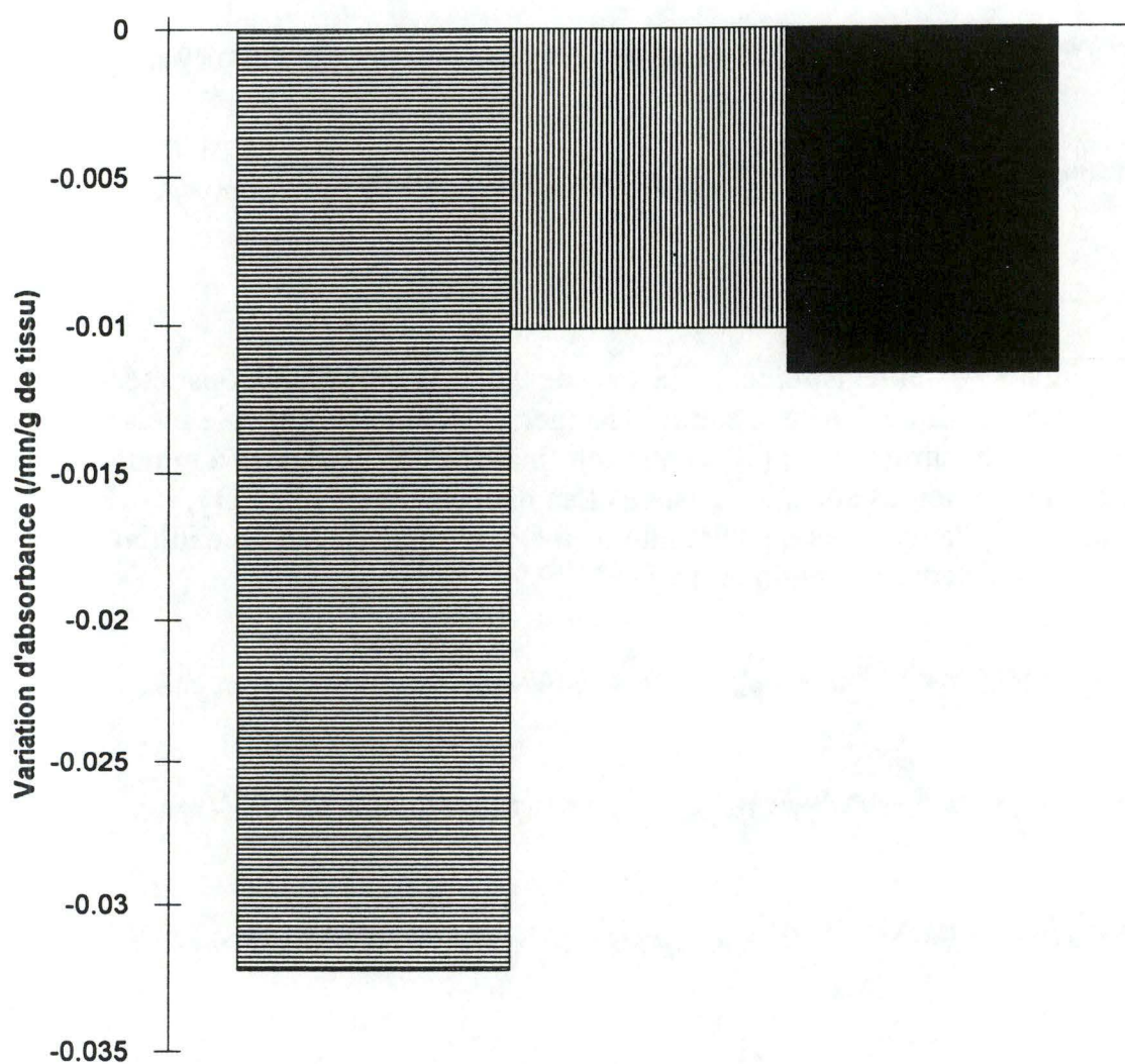
Figure 18 : Effets de l'ajout dans des extraits d'hépatopancréas de Carcinus maenas d'un inhibiteur de l'ascorbate et d'un inhibiteur des molécules possédant des groupements thiols sur l'activité réductrice des extraits d'hépatopancréas. 945 \mu l d'extraits d'hépatopancréas sont mélangés avec 52.5 \mu l de solution Tris, ou avec 52.5 \mu l du L-ascorbate oxydase (dilution dans la solution Tris pour obtenir 5 U/ml), ou avec du N-éthylmaléimide de concentration 8 mM. Les mélanges sont incubés pendant 4 mn, puis 52.5 \mu l de solution de chrome (VI) 2.5 mM est ajouté. l'absorbance à 372 nm est suivie.
