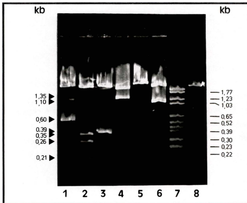
Figure 17. Analyse en gel d'agarose à 1,2% de la restriction du pG-cDAP1.1 par piste 1: Bam HI, piste 2: Hind III, piste 3: Kpn I, piste 4: Pvu I, piste 5: Xba I, piste 6: Eco RI
