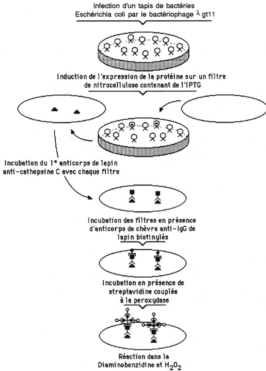
Figure 7. Criblage de la banque d'ADNc de foie de rat, \lambda gt11, au moyen d'anticorps. Dans notre cas, des anticorps polyclonaux dirigés contre la cathepsine C de foie de rat ont été utilisés.
