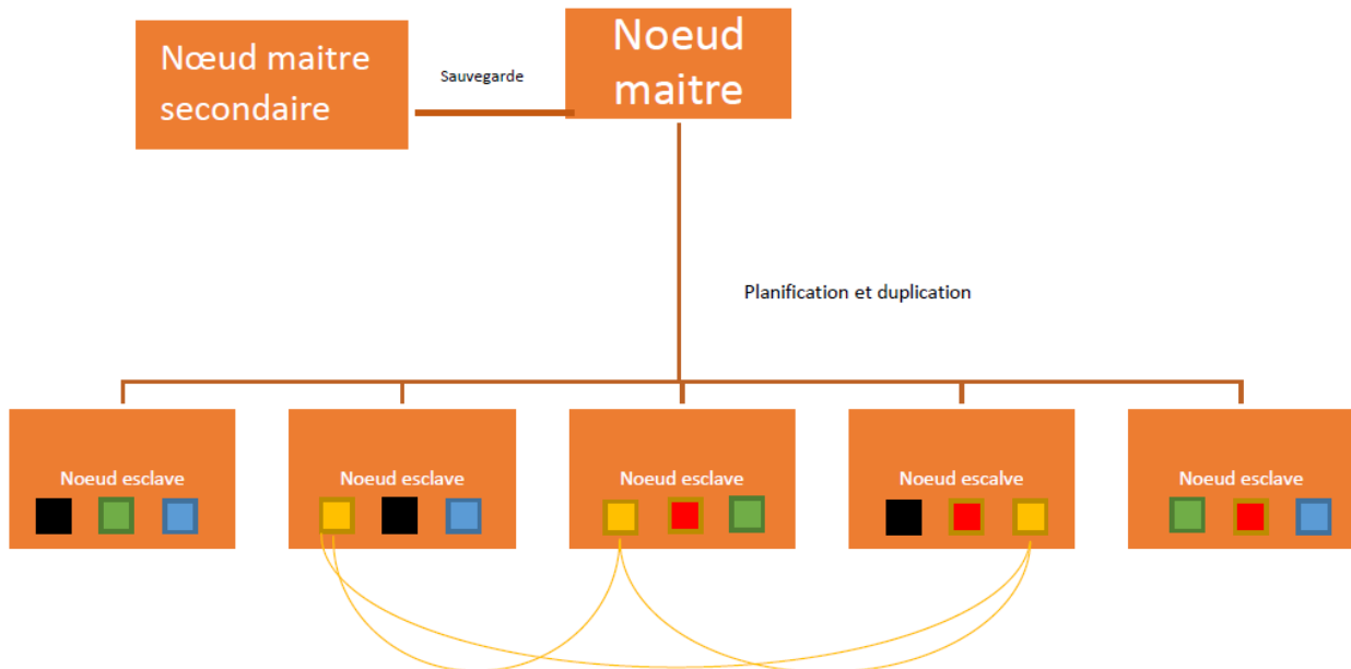
Figure 8.3 Schéma de l'architecture HDFS avec la représentation de répliquations de différents data blocs dans différents nœuds (Wikipedia contributors, 2020).
