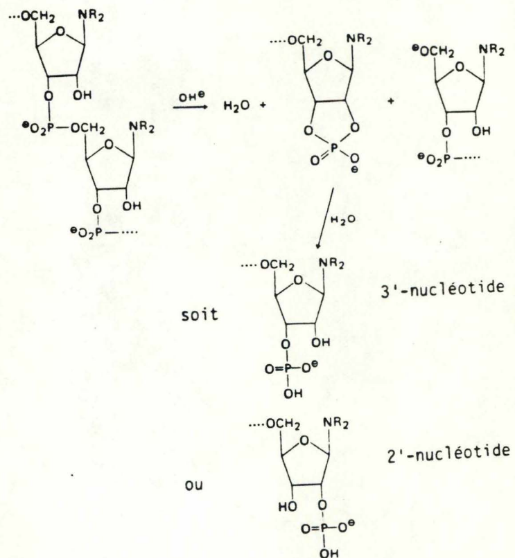
fig. 5 : L'hydrolyse alcaline de l'ARN conduit à la formation d'un intermédiaire cyclique qui forme finalement un mélange 2' ou 3'-nucléotides.
