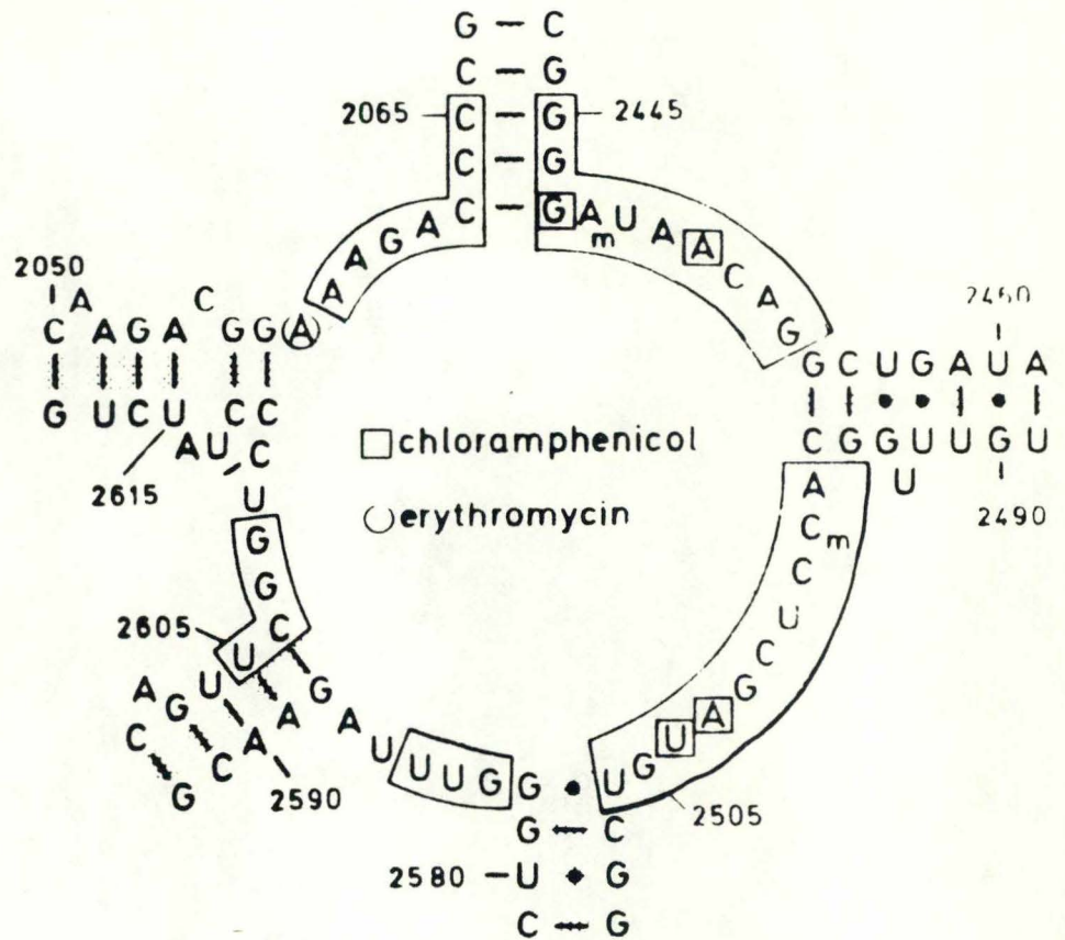
fig. 24 : Fragment de l'ARNr 23 S d' E. coli montrant les positions de modifications du nucléotide causant les résistances au chloramphénicol et à l'érythromycine. Les nucléotides modifiés ont été identifiés chez la levure et les mitochondries de mammifères et ont été transférés sur les positions correspondantes chez E. coli .
