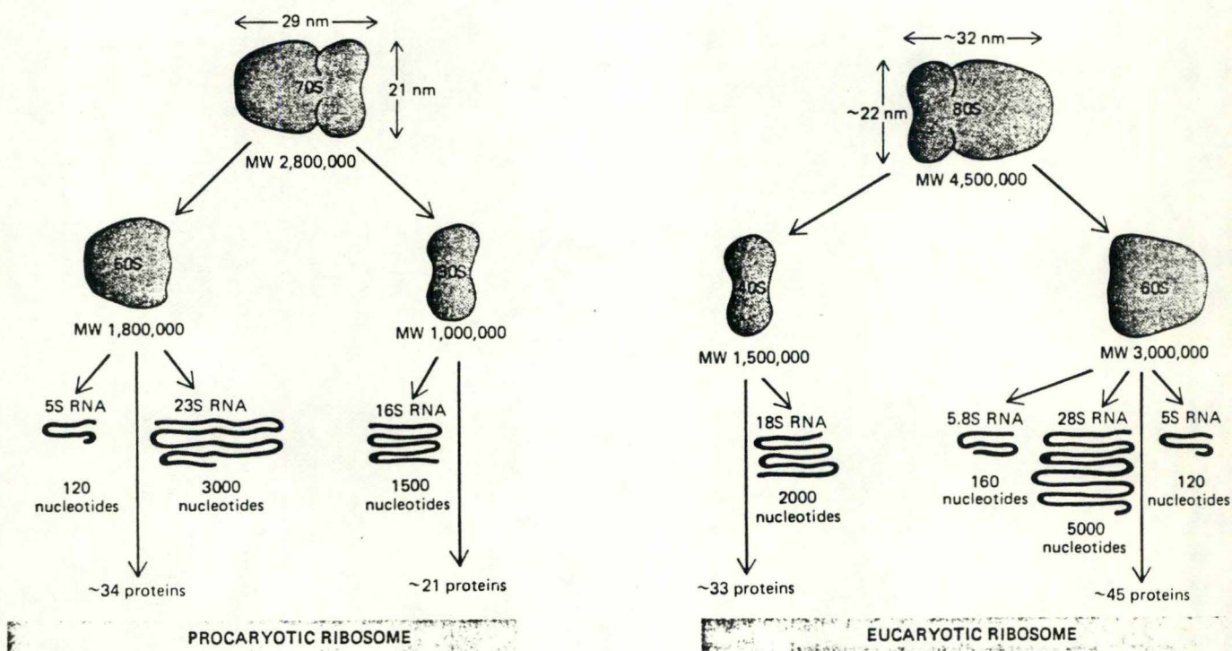
fig. 2 : Comparaison de l'organisation des ribosomes eucaryotiques et procaryotiques.
