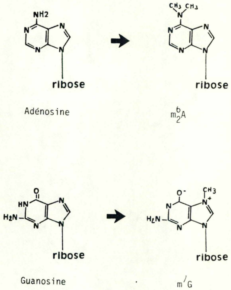
Figure 16 ----- exemple de méthylation de base dans les ARNr. comparaison avec le nucléoside non modifié correspondant.
