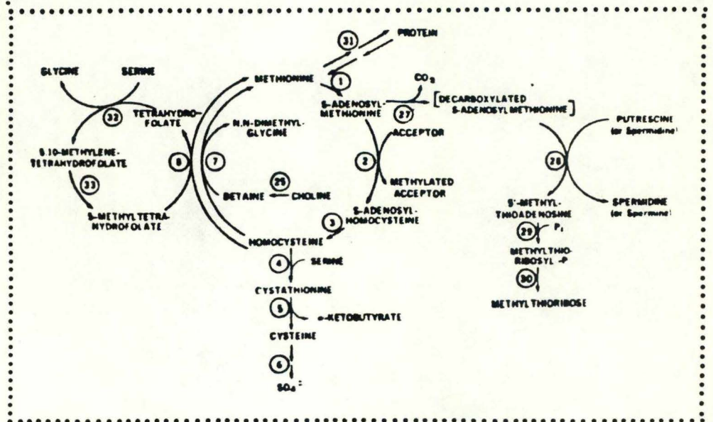
fig. 18 : Cycle biochimique du métabolisme de la méthionine. Les chiffres entourés d'un cercle représentent les enzymes catalysant les différentes réactions. L'enzyme 2 représente une méthyltransférase.
