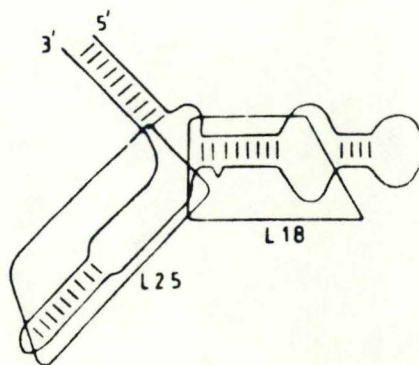
fig. 7 : Structure en "Y" de l'ARNr 5 S et sites d'interaction avec les protéines ribosomiques L18 et L25.
