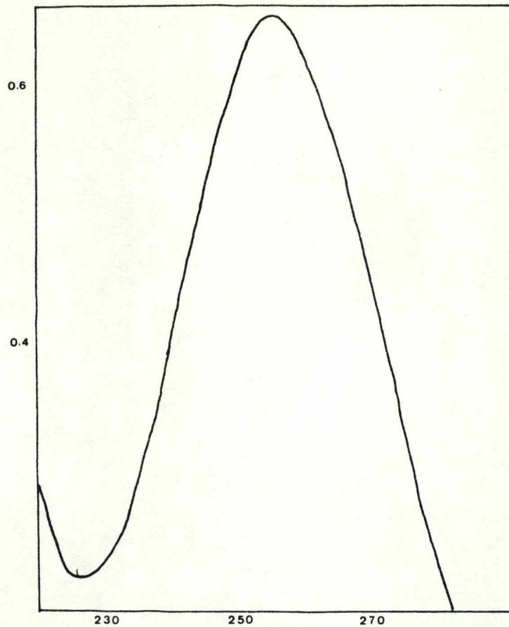
fig. 3 : Spectre UV de l'ARN total de levure
