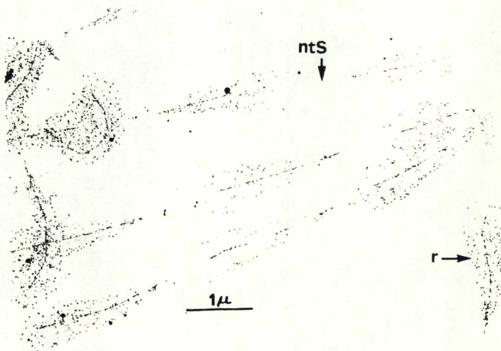
fig. 10 : Transcription de l'ADNr : image classique de l'arbre de Noël.
