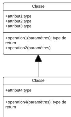
FIGURE 5.1 – Relation d'héritage dans un diagramme de classes
