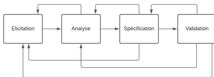
FIGURE 1.3 – Processus de développement des exigences
