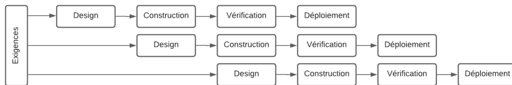
FIGURE 1.7 – Modèle incrémental
