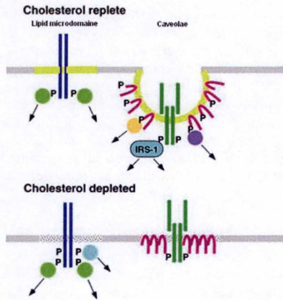
Figure 6: Schématisation de la régulation des récepteurs avant (Cholesterol replete) et après (cholesterol depleted) traitement à la M \beta CD
