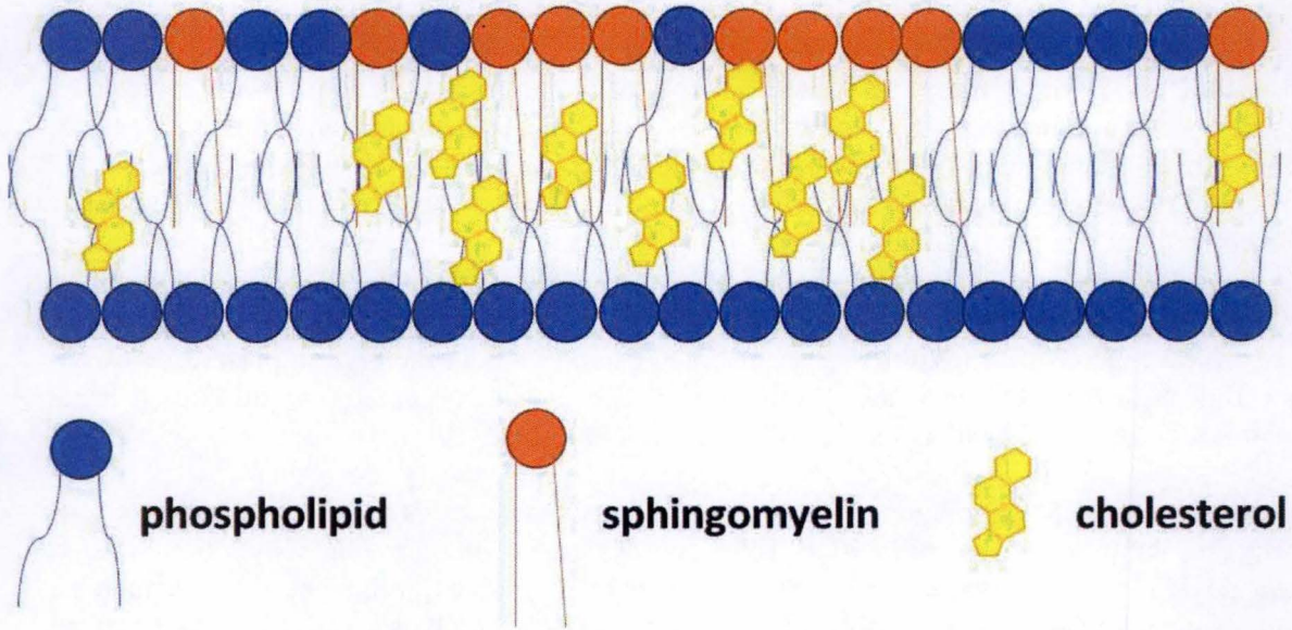
Figure 2: schématisation de la membrane plasmique avec les microdomaines lipidiques
