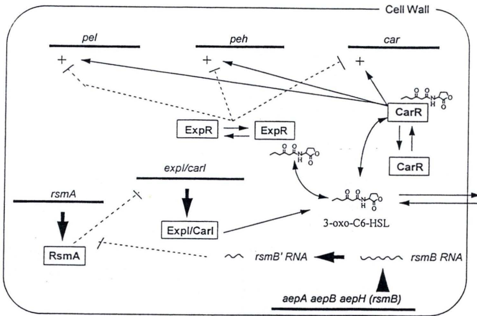
Figure 12 : Modèle de la régulation des facteurs de virulence chez E. carotovora . Les facteurs de virulence incluent la pectate lyase (Pel), la polygalacturonase (Peh) et le carbapenem qui est un antibiotique (Car) (Pierson III, Wood et al. 1999).
