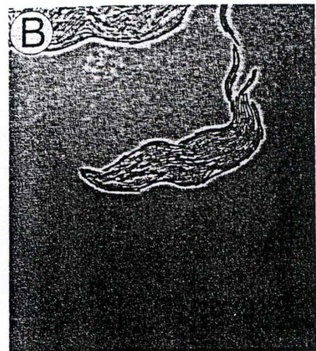
Figure 3 : Le swarming chez Proteus mirabilis (A) Cellule swarmer complètement différenciée vue par microscopie électronique (B) Mouvement de masse de cellules swarmers sur agar (Belas 1997)
