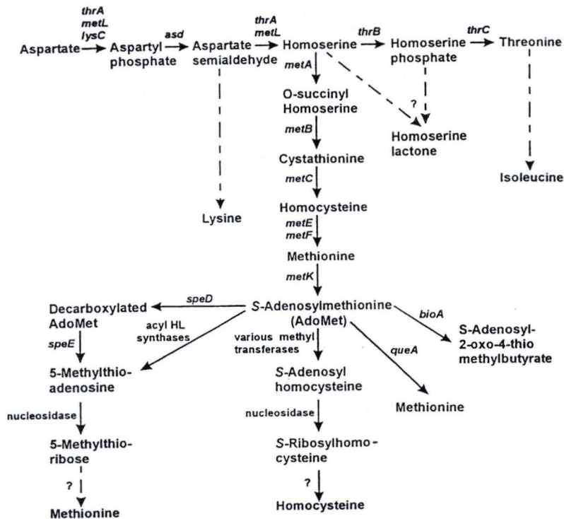
Figure 13 : Voie de synthèse biochimique méthionine-lysine-thréonine (Fuqua and Eberhard 1999).
