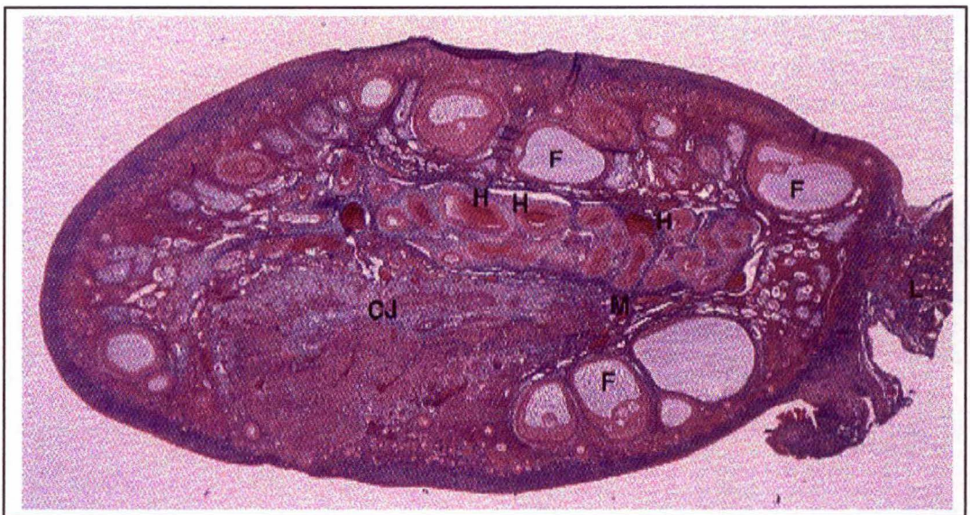
Figure 21 : Coupe transversale d'un ovaire de guenon : CJ : corps jaune, F : follicule, H : artère hélicine, L : ligament large, M : médullaire (zone centrale du stroma ovarien) (in : Histologie fonctionnelle, 1995).
