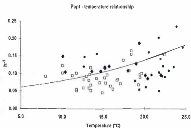
Figure 25. Relation température (°C) – P_{opt} ( h^{-1} ) d'après Descy et al. (1994) avec superposition des points de notre étude (représentés par les losanges).
