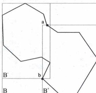
FIG. 4.14 – La plus petite AABB d'un ensemble de primitives englobe les plus petites AABB des sous-ensembles des partitions de l'ensemble (2D)
