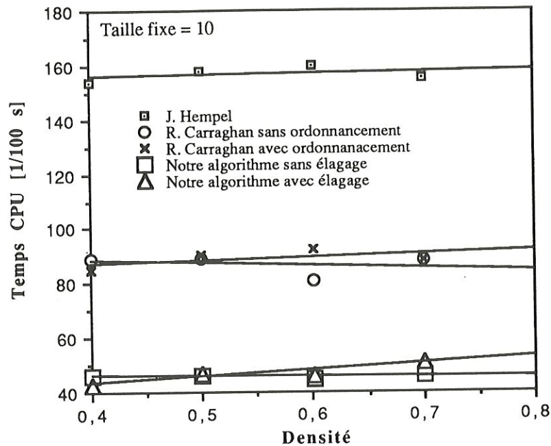
Figure 6.1: Temps d'exécution en fonction de la densité
