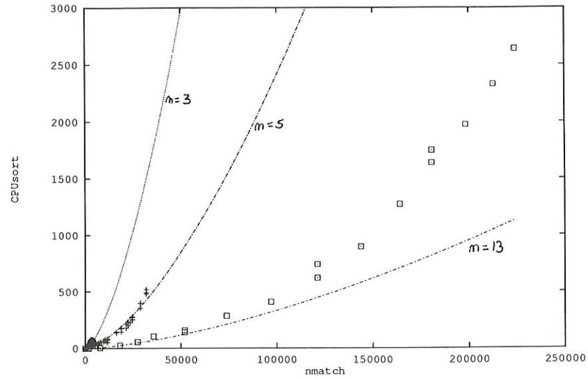
Figure 6.19: CPU sort en fonction de n match pour deep>1
