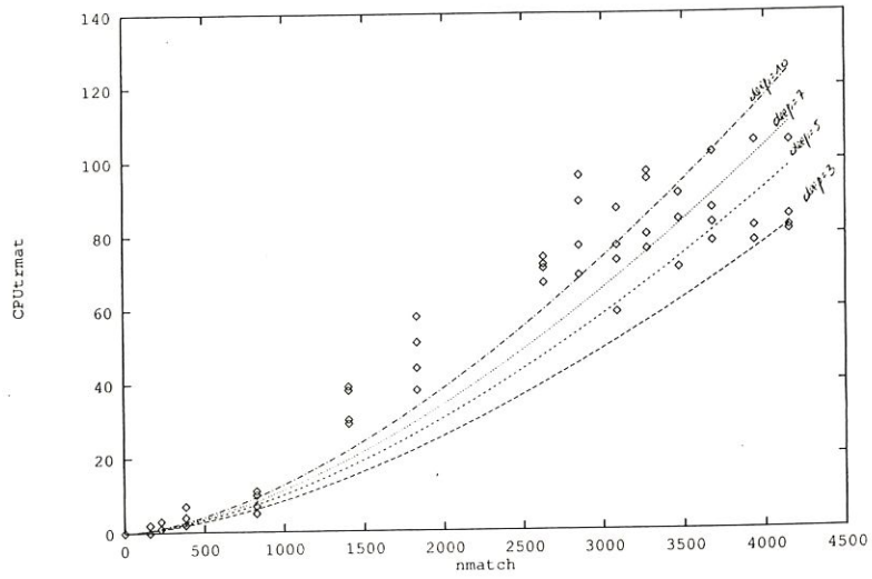
Figure 6.16: CPU trmat en fonction de n match pour n=3 et deep>1
