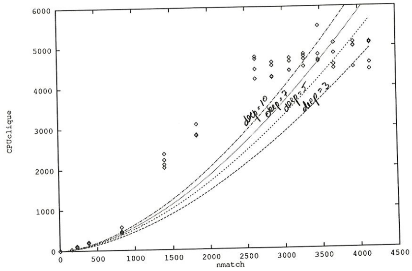
Figure 6.21: CPUclique pour n=3 et deep>1
