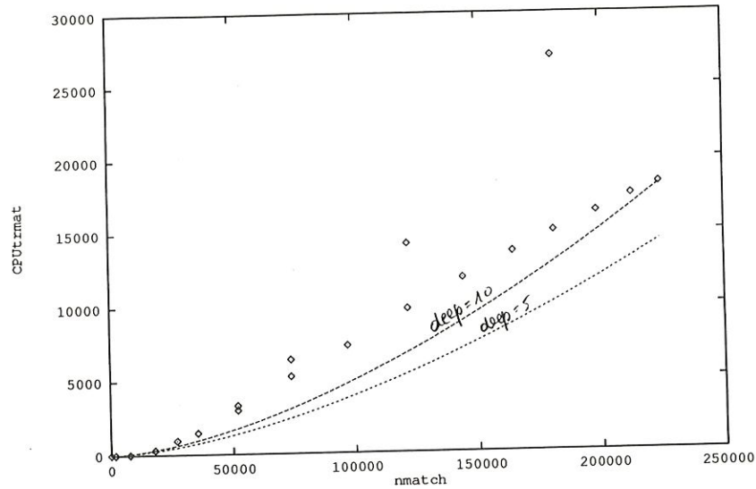
Figure 6.18: CPU trmat en fonction de nmatch pour n=13 et deep>1
