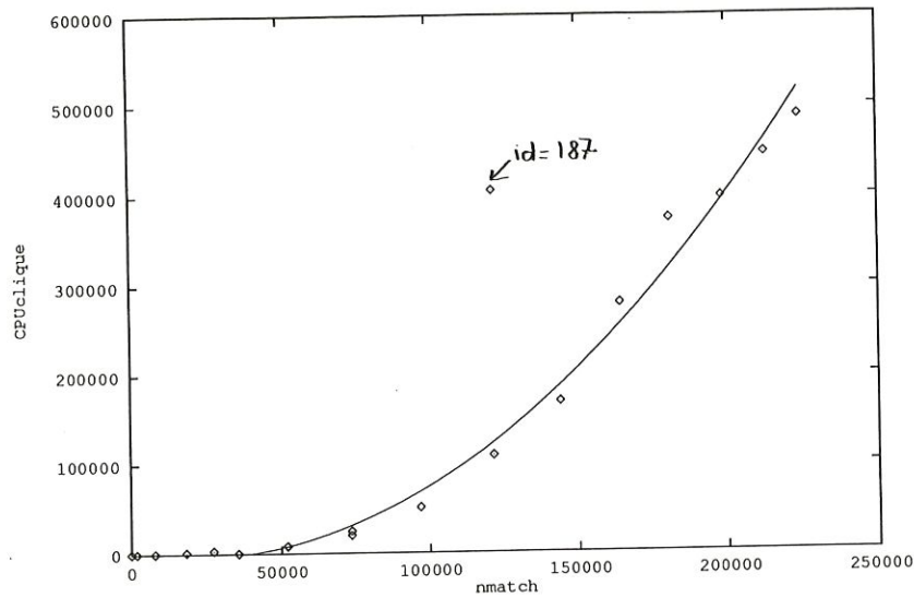
Figure 6.26: Le CPUclique en fonction de nmatch pour n=13 et deep>1
