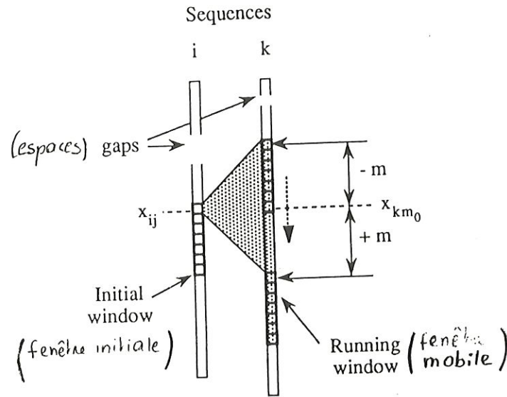
Figure 2.1: Le balayage des séquences
