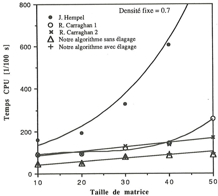
Figure 6.3: Temps d'exécution en fonction de la taille de la matrice
