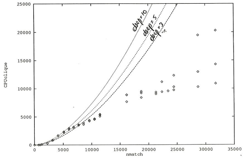
Figure 6.22: CPUclique pour n=5 et deep>1
