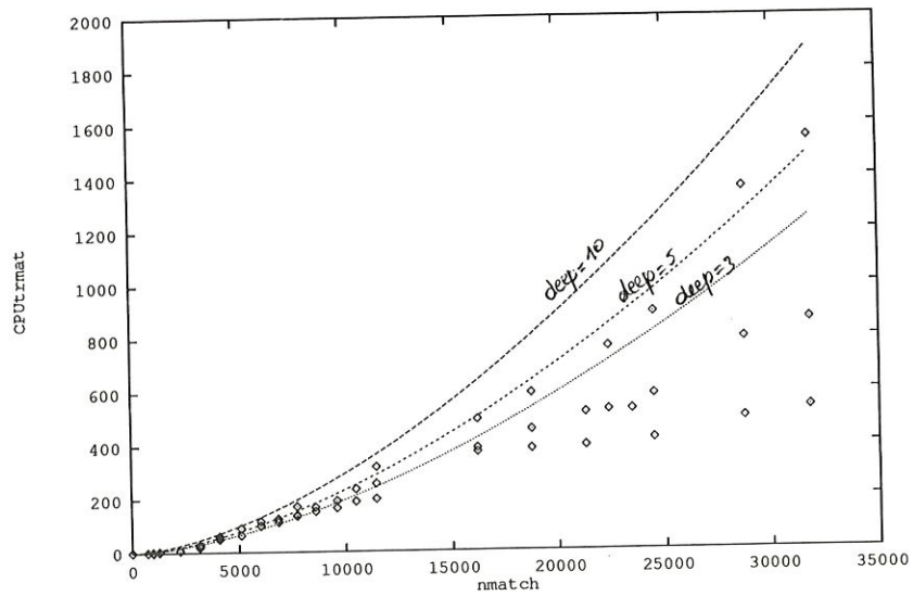
Figure 6.17: CPU trmat en fonction de n match pour n=5 et deep>1
