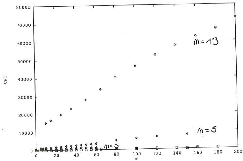
Figure 6.8: Les différents CPU pour tous les tests avec deep = 1
