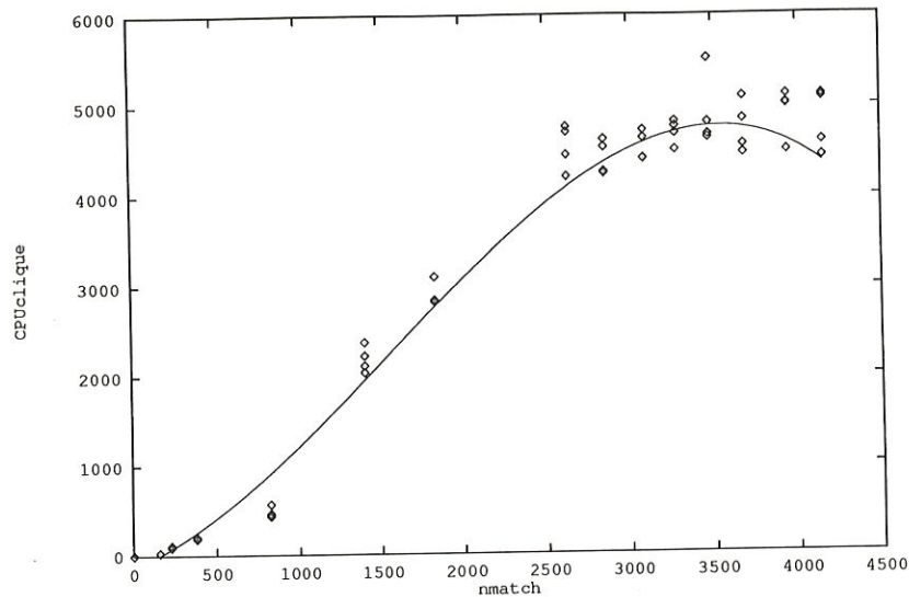
Figure 6.24: Le CPUclique en fonction de nmatch pour n=3 et deep>1
