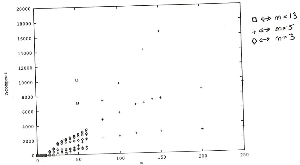
Figure 6.27: Nombre de matches complets en fonction de m.
