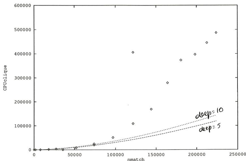
Figure 6.23: CPUclique pour n=13 et deep>1
