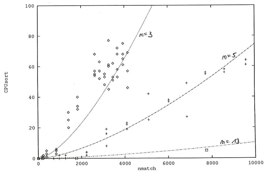
Figure 6.20: CPU sort en fonction de n match pour deep > 1
