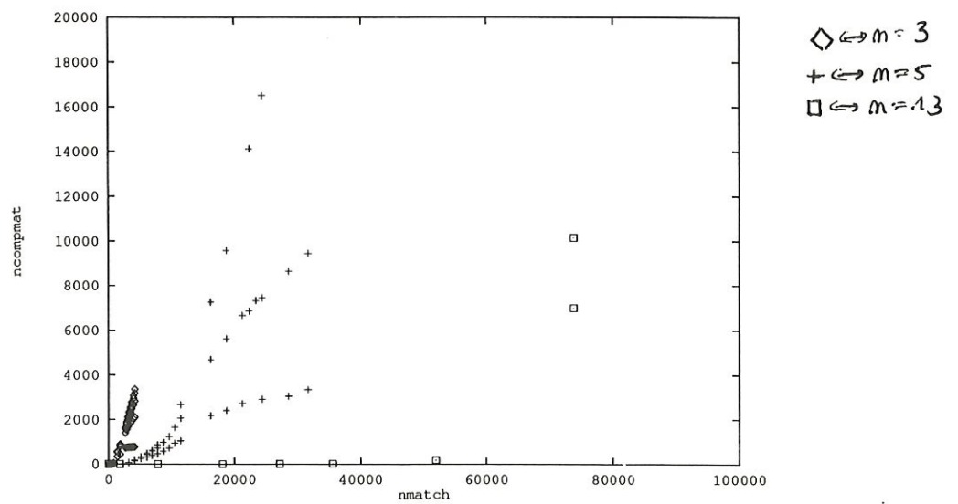
Figure 6.29: Nombre de matches complets en fonction de nmatch.
