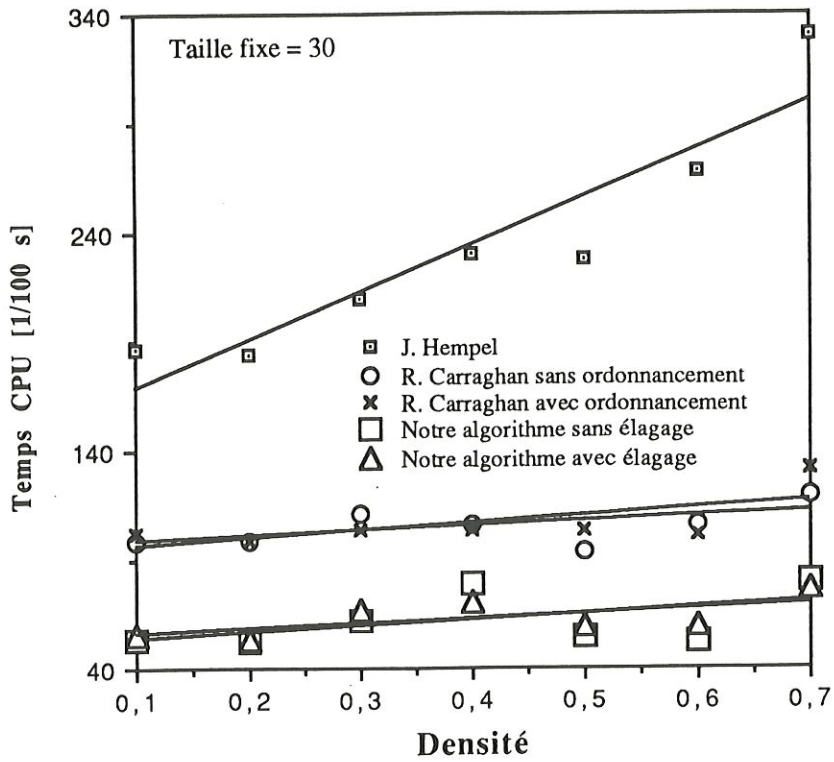
Figure 6.2: Temps d'exécution en fonction de la densité de la matrice
