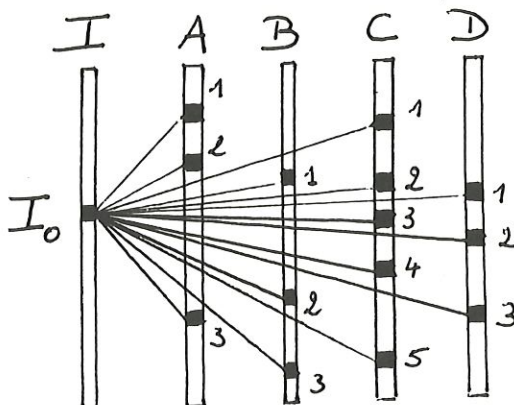
Figure 5.2: Exemple pour l'algorithme "efficace".
