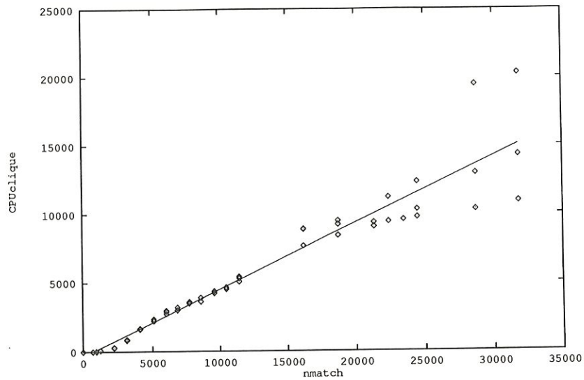
Figure 6.25: Le CPUclique en fonction de nmatch pour n=5 et deep>1
