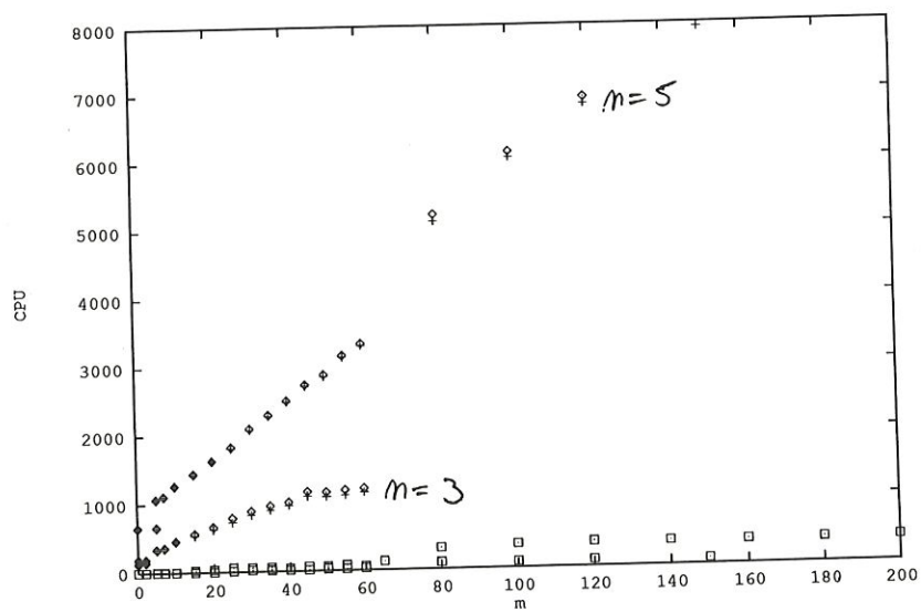
Figure 6.9: Les différents CPU pour tous les tests avec deep = 1
