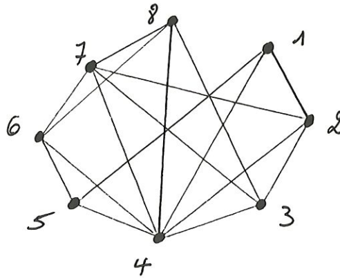
Figure 5.1: Le graphe G = (X \cup U) avec X = \{1, 2, 3, 4, 5, 6, 7, 8\} .
