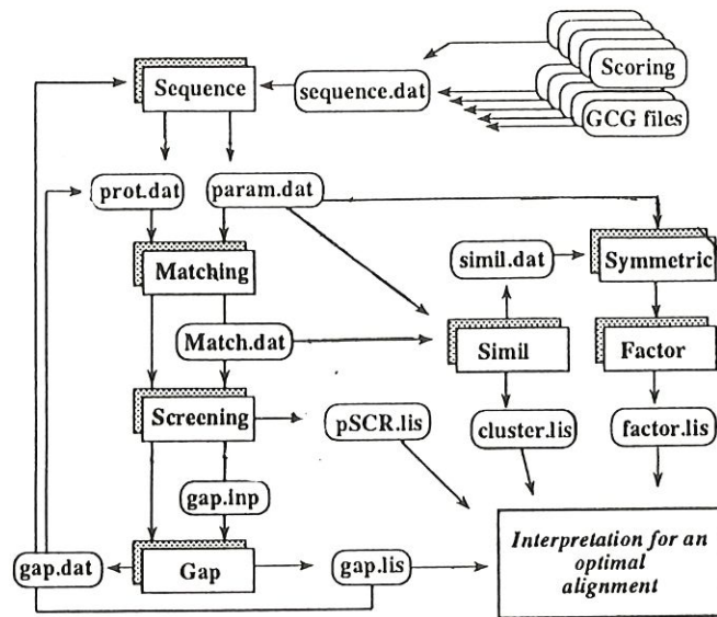
Figure 2.4: Algorithme de l'alignement multiple de E. Depiereux et E. Feytmans.
