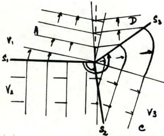
Figure 18 . Interaction avec un point triple (ang 1 < 180 et ang 2 ≥ 180°)
