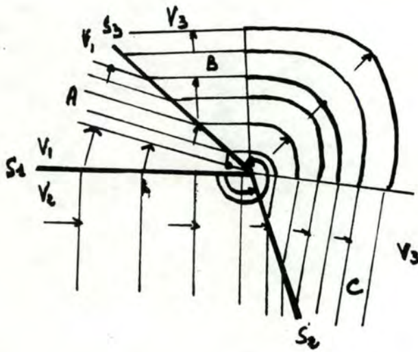
Figure 18 . Interaction avec un point triple (ang 1 < 180 et ang 2 ≥ 180°)
