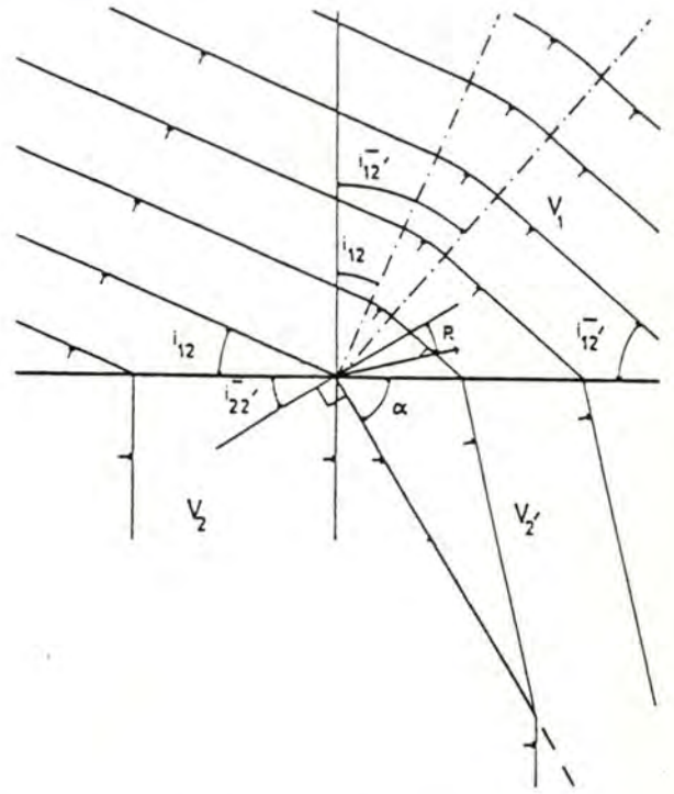
Figure 23. Interaction avec un point triple ( V_1 < V_2' < V_2 ). L'onde principale se propage dans le milieu V_2 (ang 1 < 180, ang 2 = 180 degrés)(réf. [3] )
