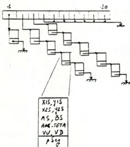
Figure 26 . Ensemble des listes chaînées attachées au modèle de terrain de la figure .
