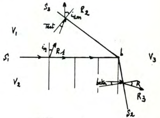
Figure 18 . Interaction avec un point triple (ang 1 < 180 et ang 2 ≥ 180°)
