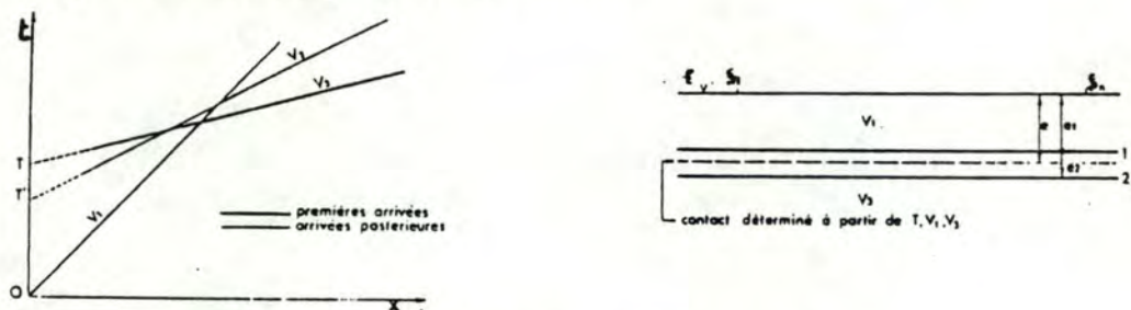
Figure 9. Phénomène de disparition d'un terrain mince (réf. [1]).
