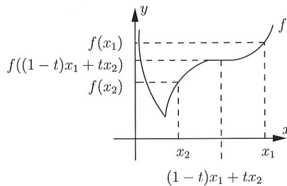
FIG. 1.1 – Illustration d'une fonction quasiconvexe
