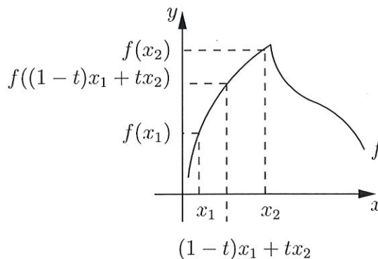
FIG. 1.4 – Illustration d’une fonction strictement quasiconcave
