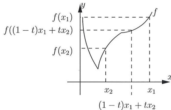
FIG. 1.3 – Illustration d'une fonction strictement quasiconvexe
