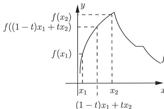
FIG. 1.2 – Illustration d'une fonction quasiconcave
