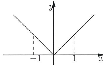
FIG. 2.1 - f(x) = |x|
