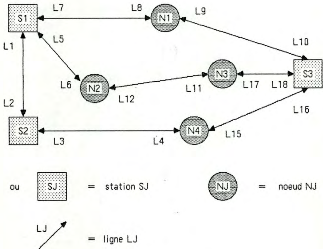
fig 1.3 Exemple de topologie n°1
