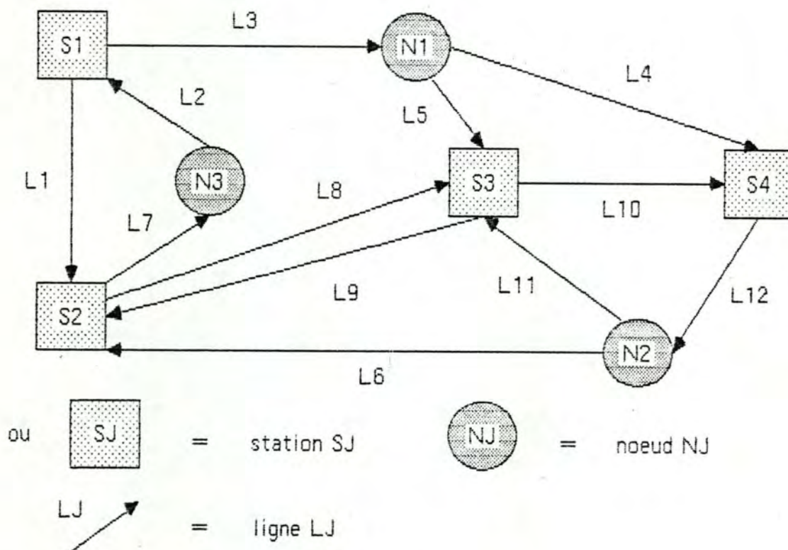
fig 1.4 Exemple de topologie n°2
