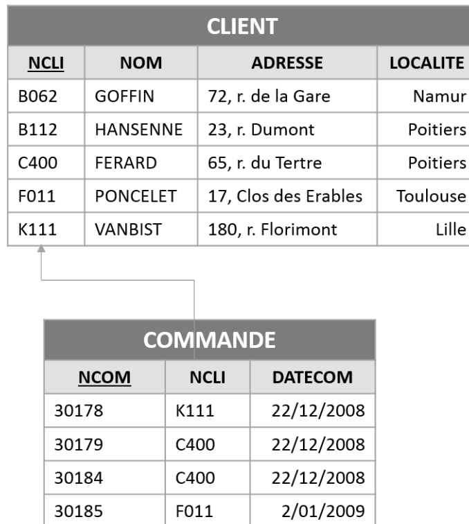
FIGURE 1.2 – Modèle relationnel classique
