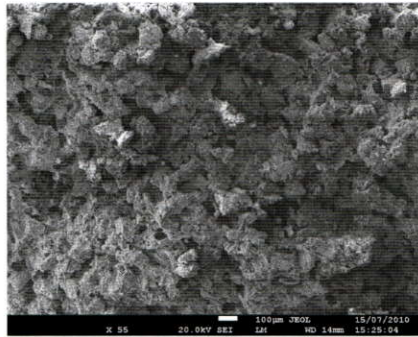
Fig. 24.- Image MEB d'un mortier jaune. © Aline Wilmet.
