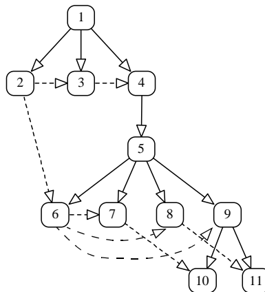
c) The SDG.
