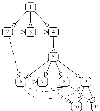
c) The SDG.
